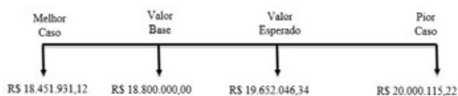
Figura 1: Cálculo do espectro do gerenciamento de riscos
