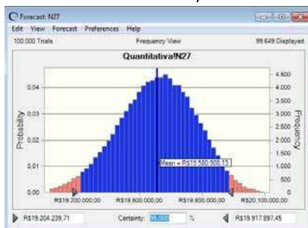
Figura 2: Gráfico resultante da simulação de Monte Carlo com Crystal Ball.
