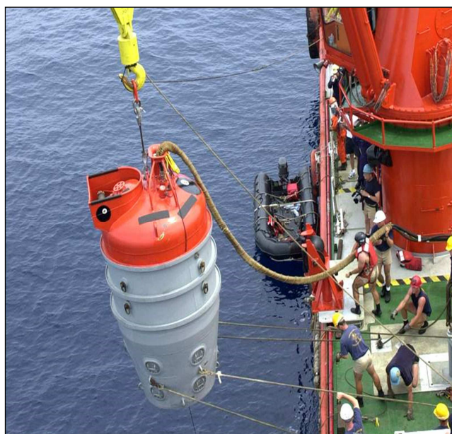
FIGURA 6 - Representação gráfica do sino tipo McCann . Fonte: Revista O Periscópio, 2006, p. 78.
